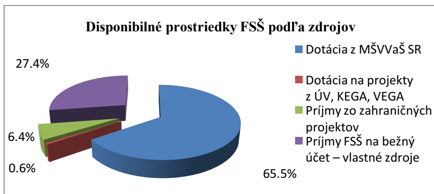
Graf č. 9.1 Disponibilné zdroje fakulty celkom v % za rok 2015
