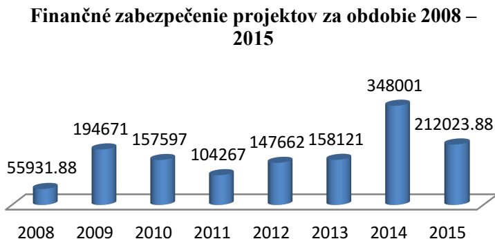
Graf. 2 Finančné zabezpečenie výskumných a kultúrno-edukačných projektov riešených FSS UKF (okrem inštitucionálnych projektov)
