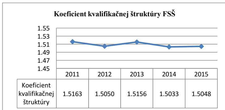
Graf č. 9.6 Vývoj koeficientu kvalifikačnej štruktúry pedagógov FŠŠ
