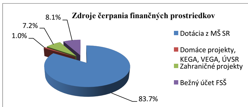
Graf č. 9.3 Podiel jednotlivých zdrojov na financovaní nákladov FSS v roku 2015
