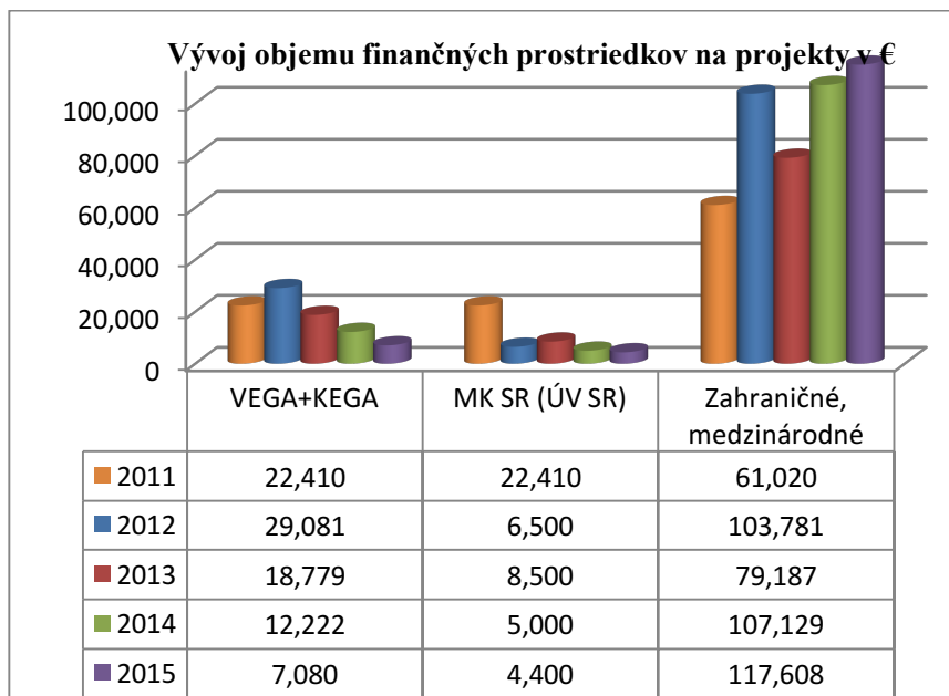
Graf. č. 9.2 Vývoj objemu finančných prostriedkov pridelených na úspešné projekty FSŠ
