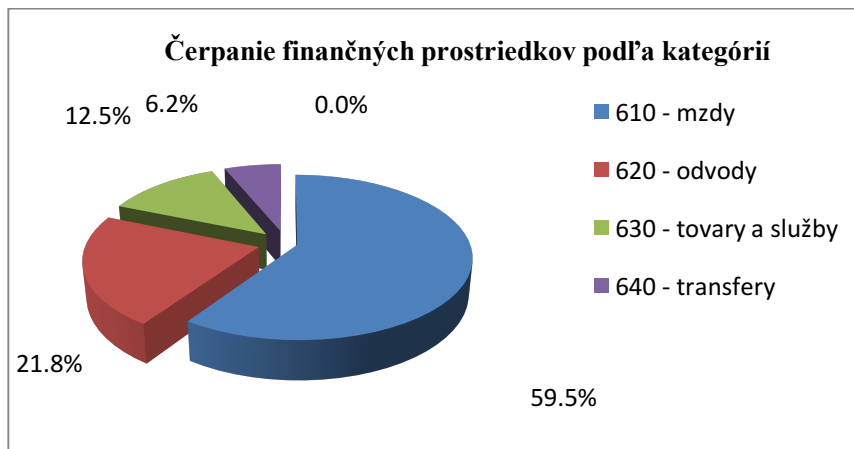
Graf č.10.4 Čerpanie finančných prostriedkov FŠŠ podľa kategórií v roku 2015
